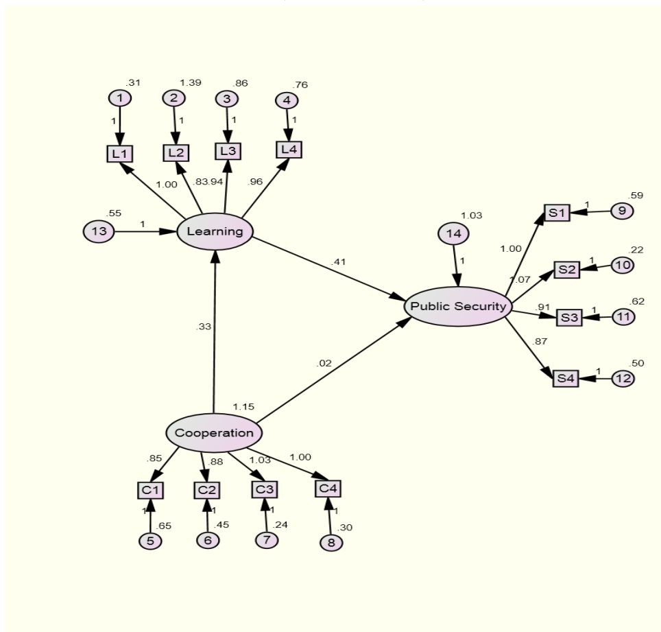
نمودار ۲. مدل معادلات ساختاری در فضای AMOS
