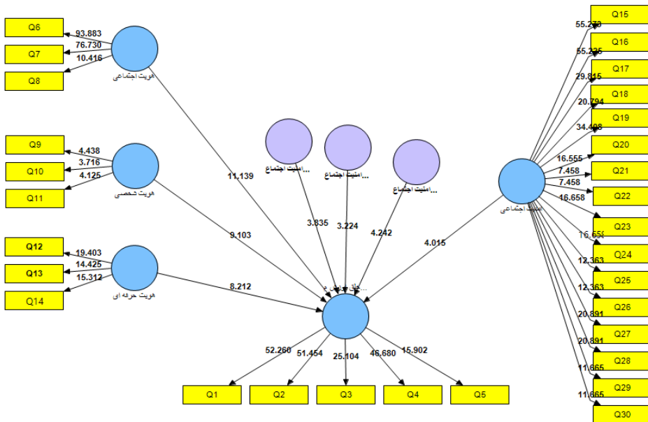
شکل ۳: خروجی نرم افزار PLS مربوط به آماره t
