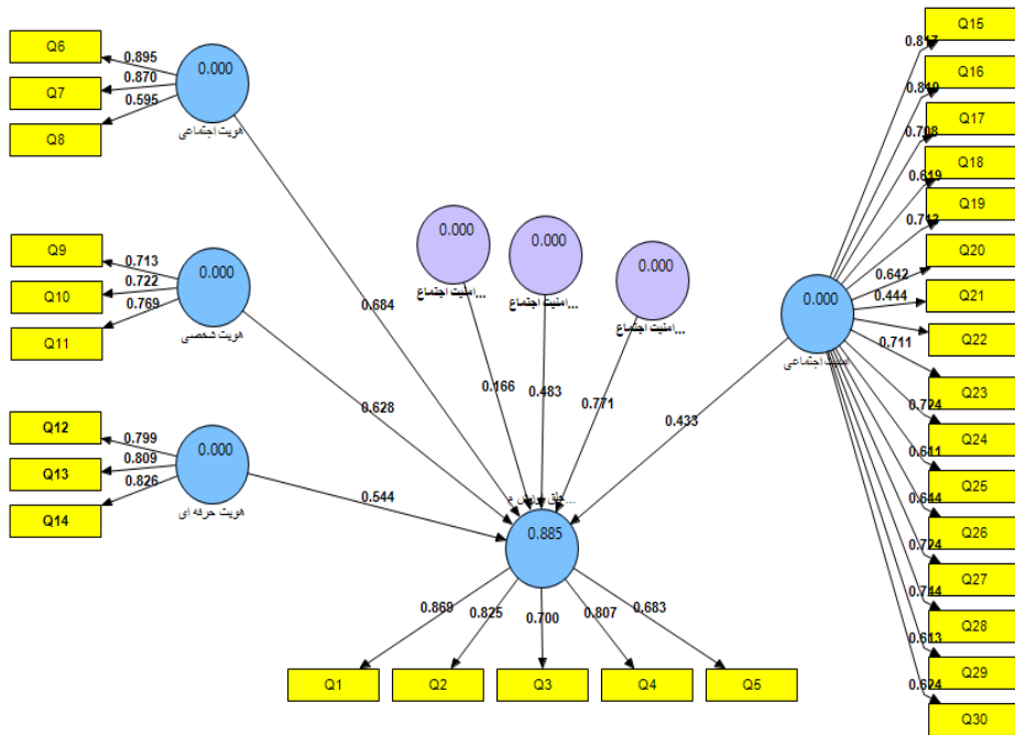
شکل ۲: خروجی نرم افزار PLS مربوط به ضرایب مسیر
